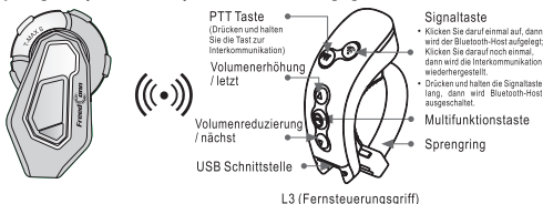
L3 (Fernsteuerungsgriff)
